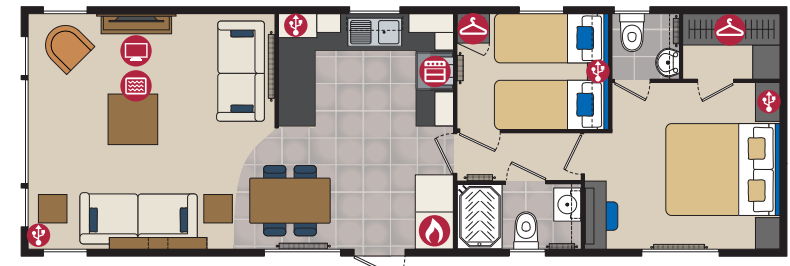
40ft x 13ft - 2 bedroom
