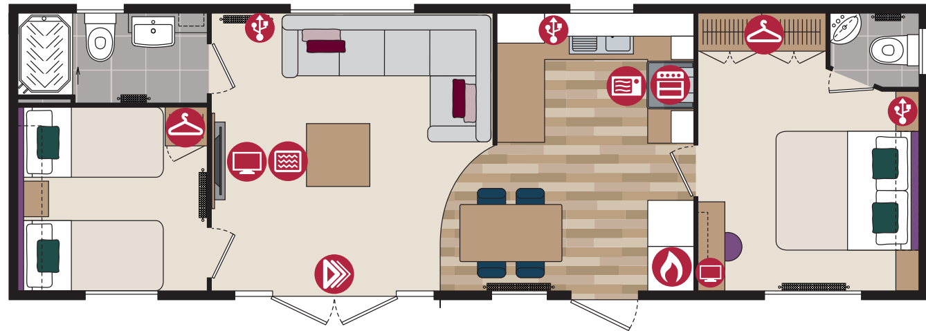
38ft x 12ft - 2 bedroom (Centre Lounge)
