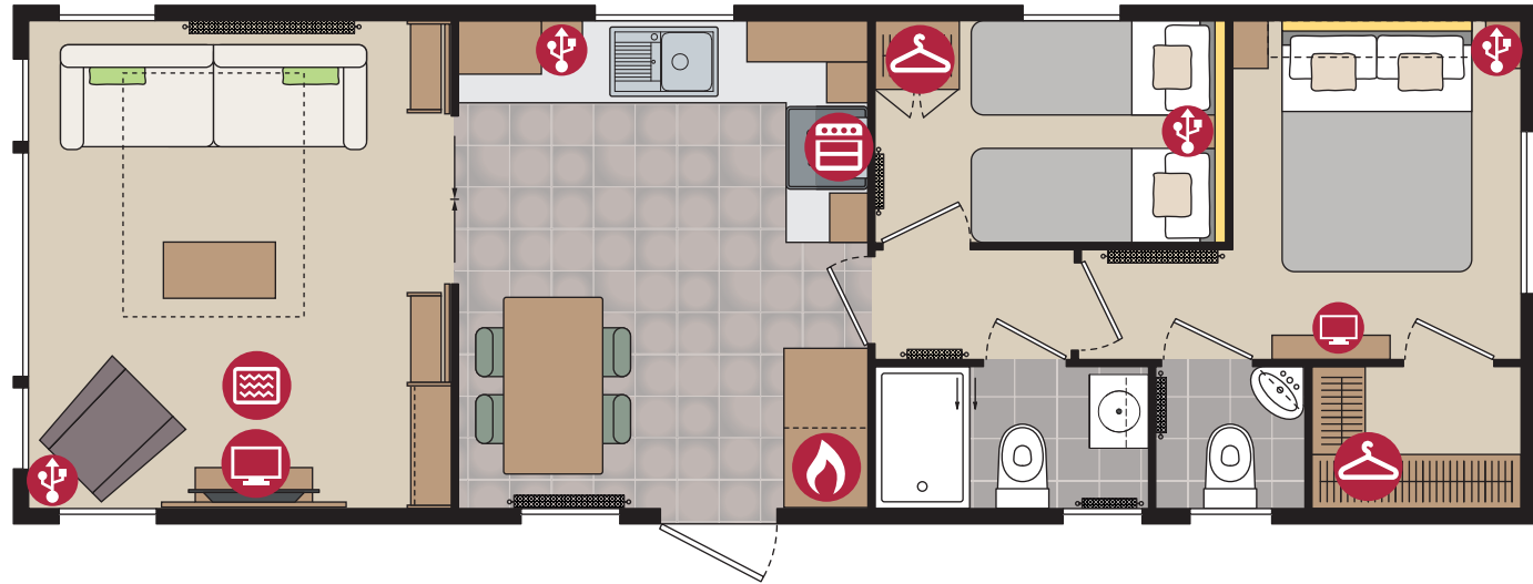
36ft x 12ft - 2 bedroom
