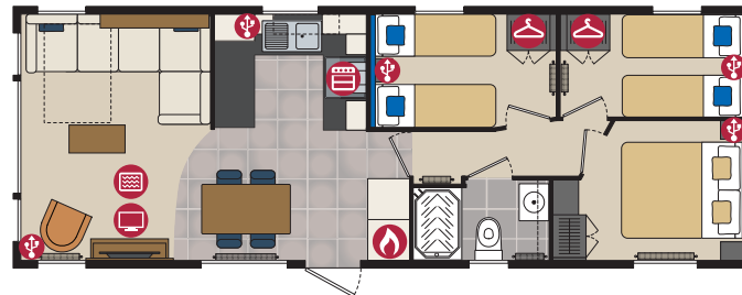
35ft x 12ft - 3 bedroom
